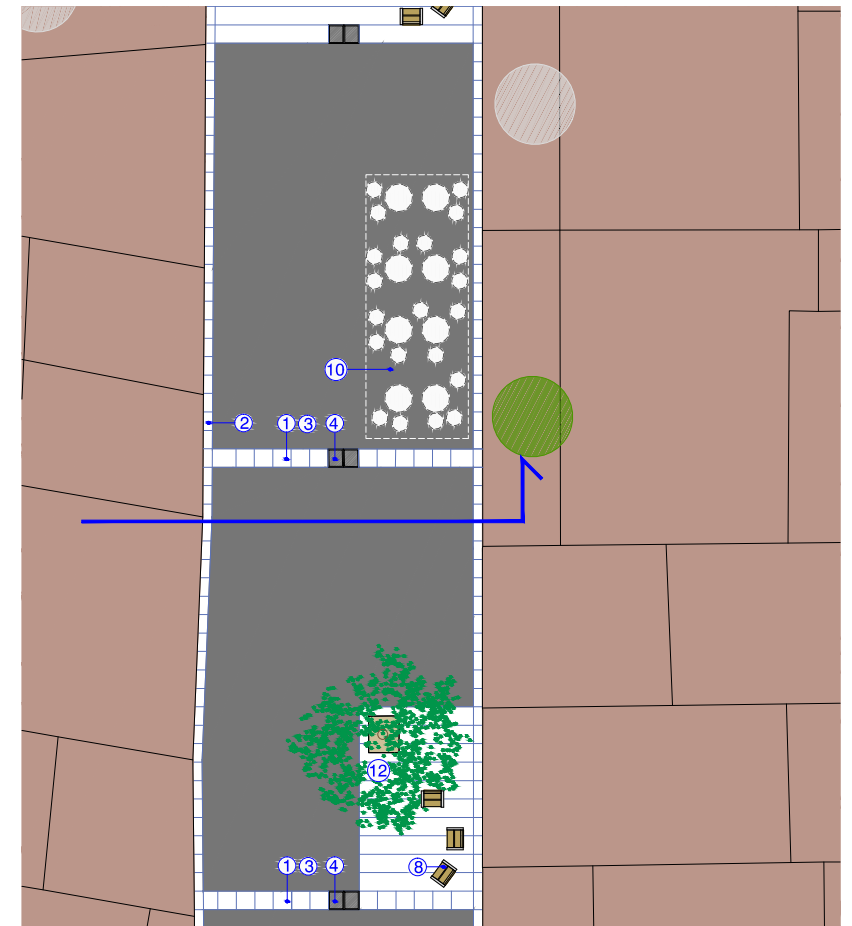
PL.TIPUS-2. ÀMBIT CENTRAL . e.: 1/150
