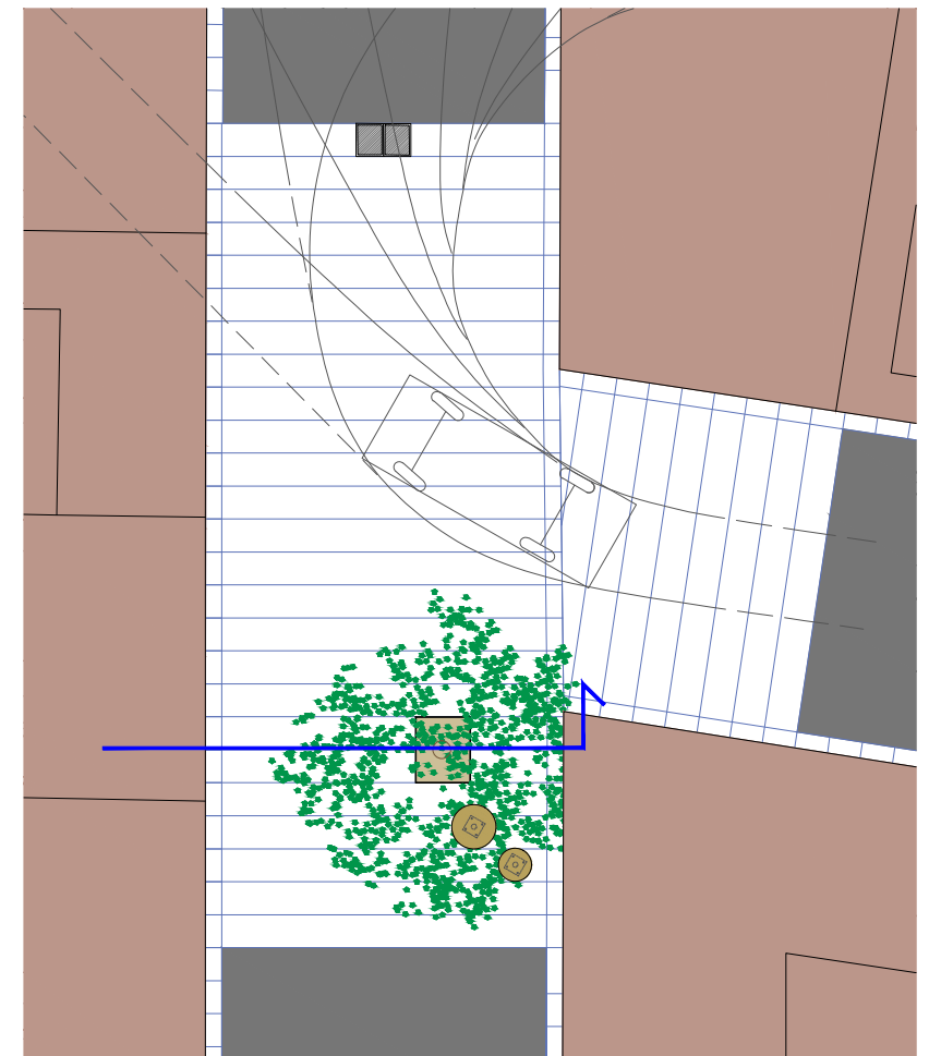
PL.TIPUS-1. ZONES DE CREUAMENT I GIR DE COTXES. e.: 1/150
