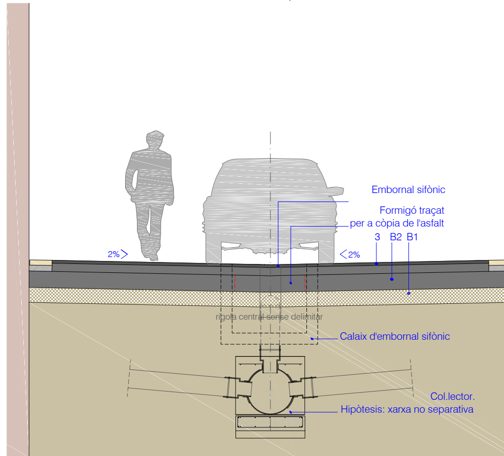
SECCIÓ TIPUS-2. PAVIMENT D'ASFALT. e.: 1/50
